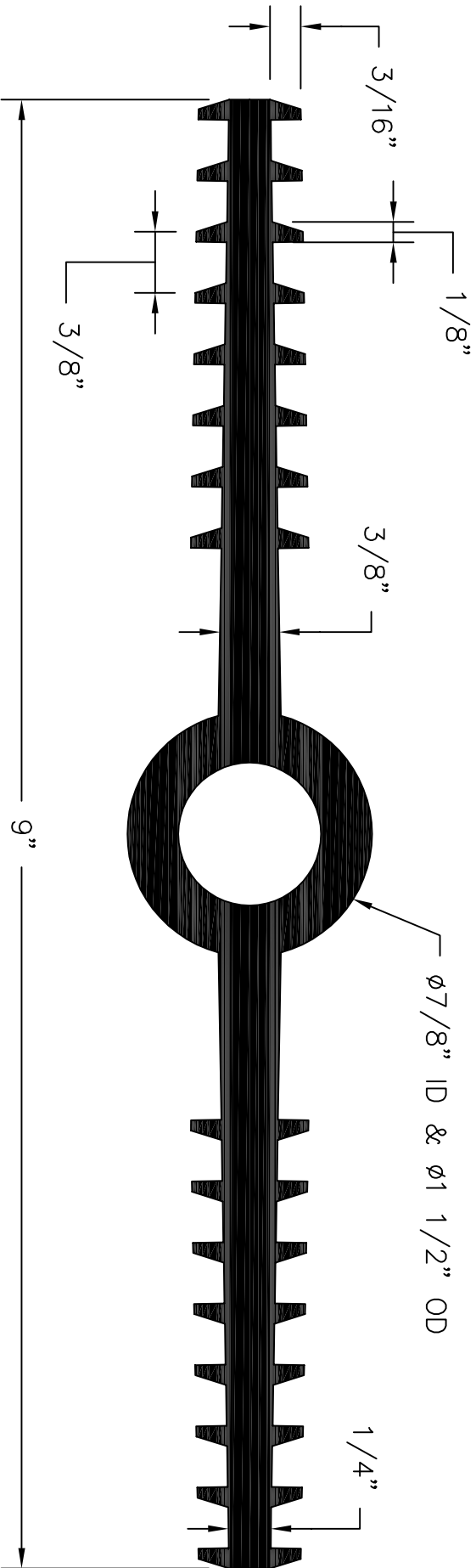
696 PROFILE SCALE: 1" = 1"
